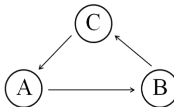
Figura 1: Tripla de Condorcet.
